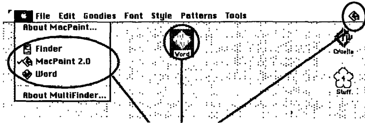
شكل (٥-٦) : ثلاث طرق لاختيار فتح تطبيقات في MultiFinder .
